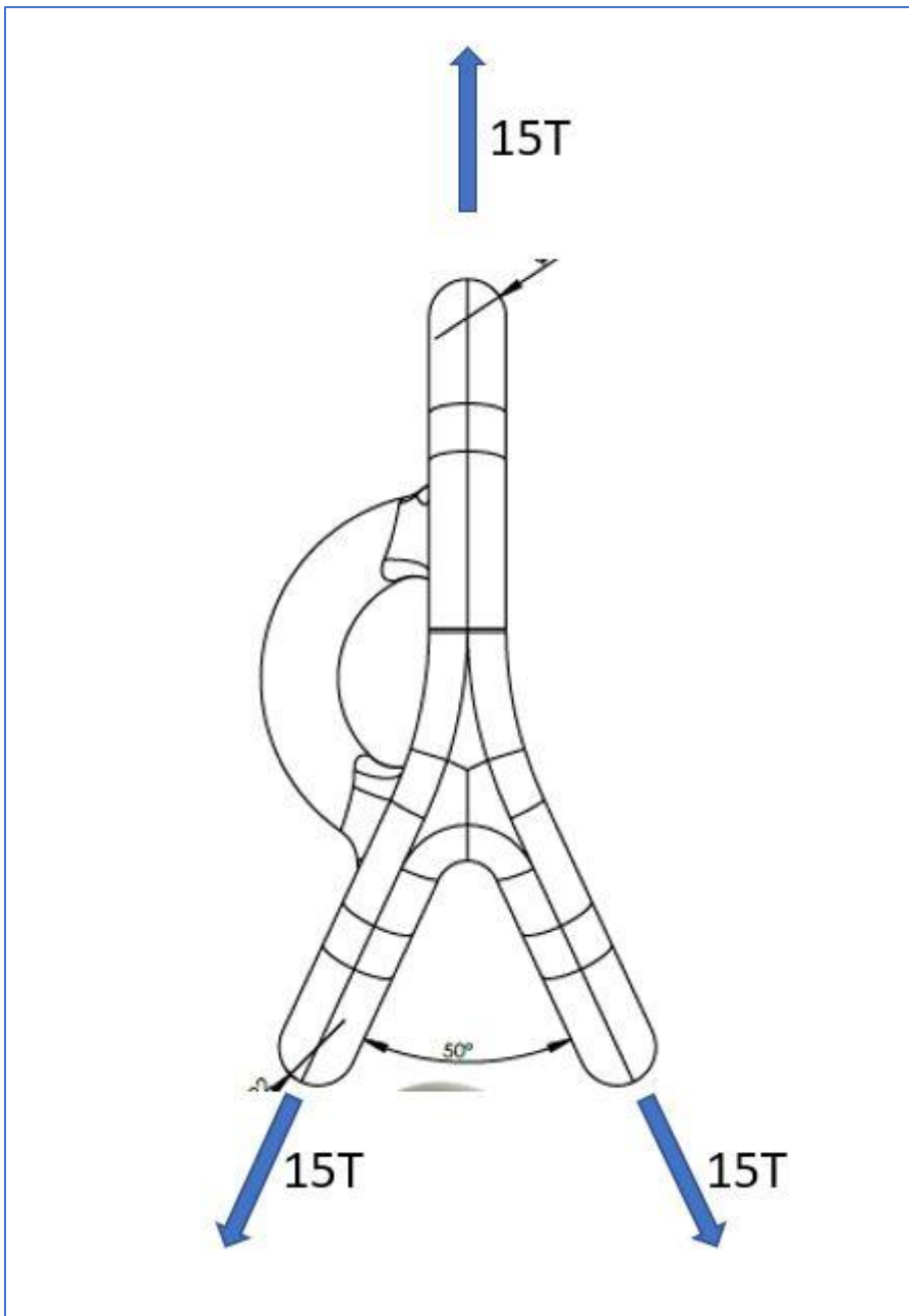
Figur 4 Tillatte laster mot seigmann
